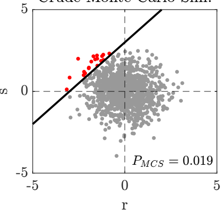
Crude Monte Carlo Sim.
